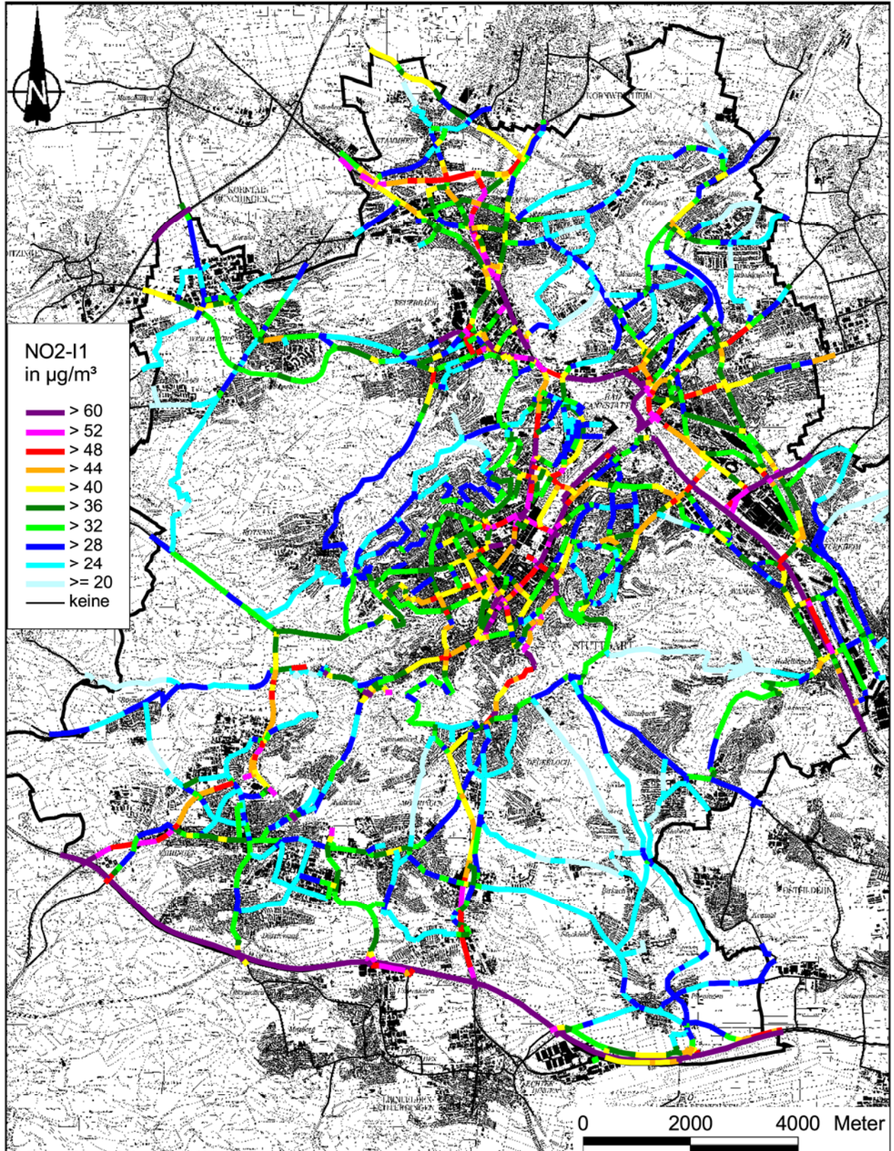
Abb. A2.2: NO 2 -Immission (Jahresmittelwert) für die Maßnahme M1 im Jahr 2010 für das Straßennetz im Stadtgebiet von Stuttgart
