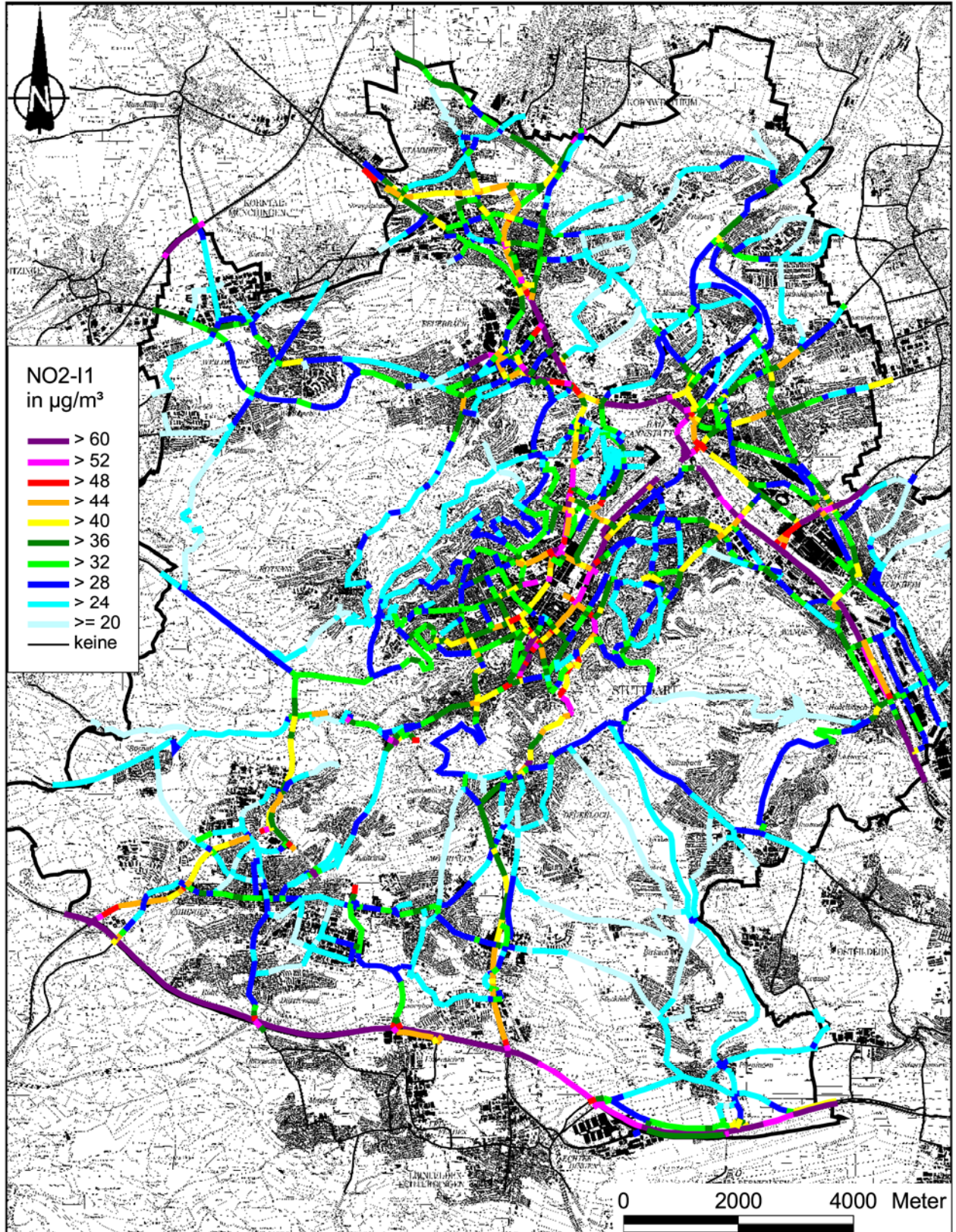
Abb. A2.3: NO 2 -Immission (Jahresmittelwert) für die Maßnahme M1+M2, Stufe 3 im Jahr 2012 für das Straßennetz im Stadtgebiet von Stuttgart
