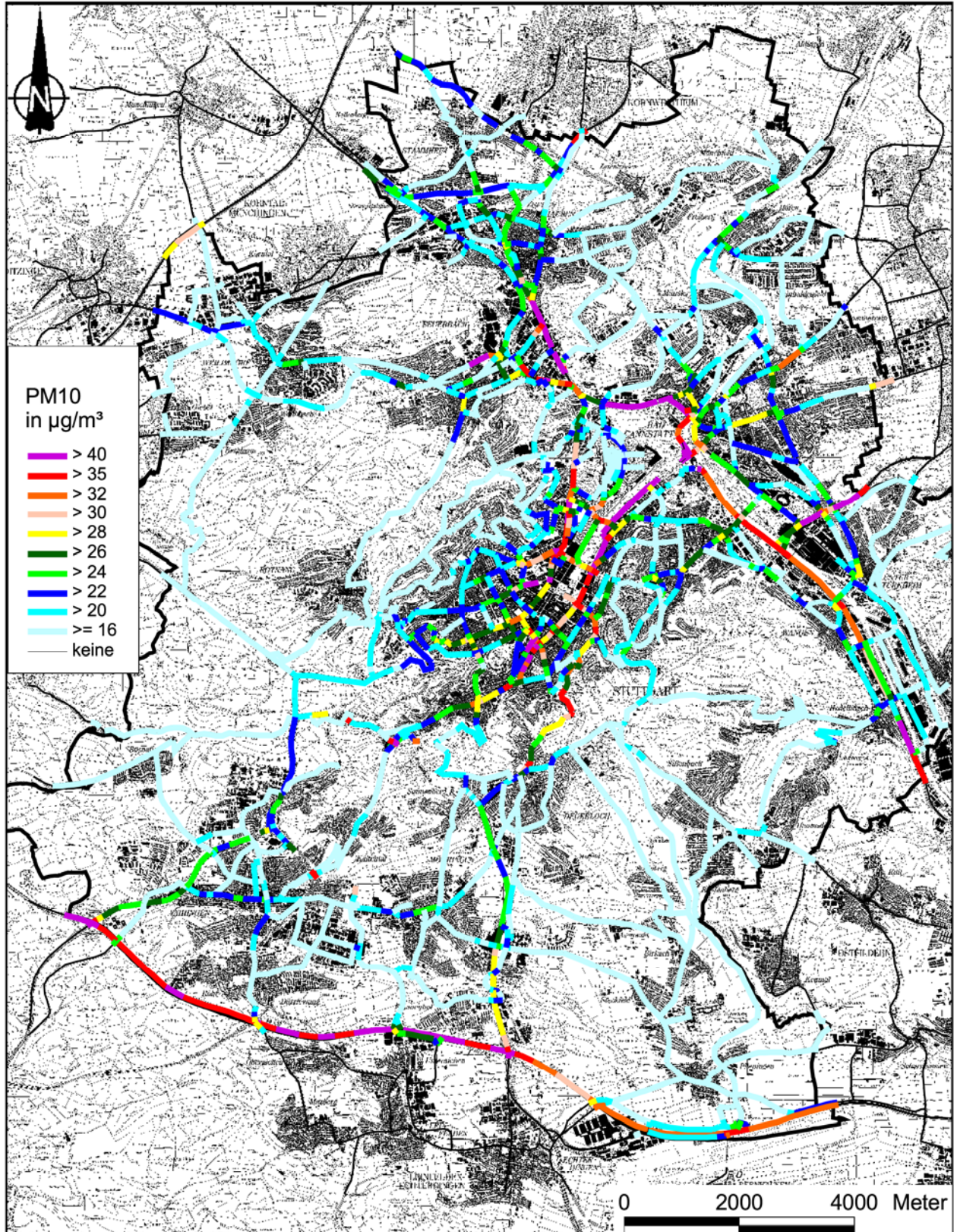
Abb. A2.5: PM10-Immission (Jahresmittelwert) für die Maßnahme M1 im Jahr 2010 für das Straßennetz im Stadtgebiet von Stuttgart
