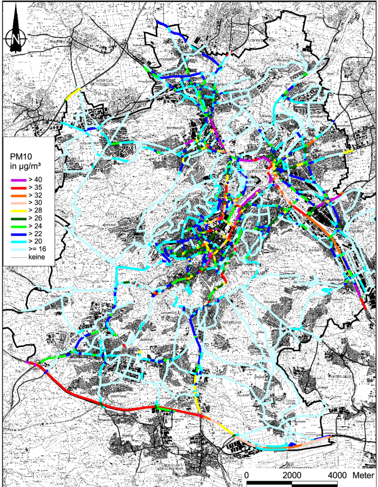
Abb. A2.6: PM10-Immission (Jahresmittelwert) für die Maßnahme M1+M2, Stufe 3 im Jahr 2012 für das Straßennetz im Stadtgebiet von Stuttgart
