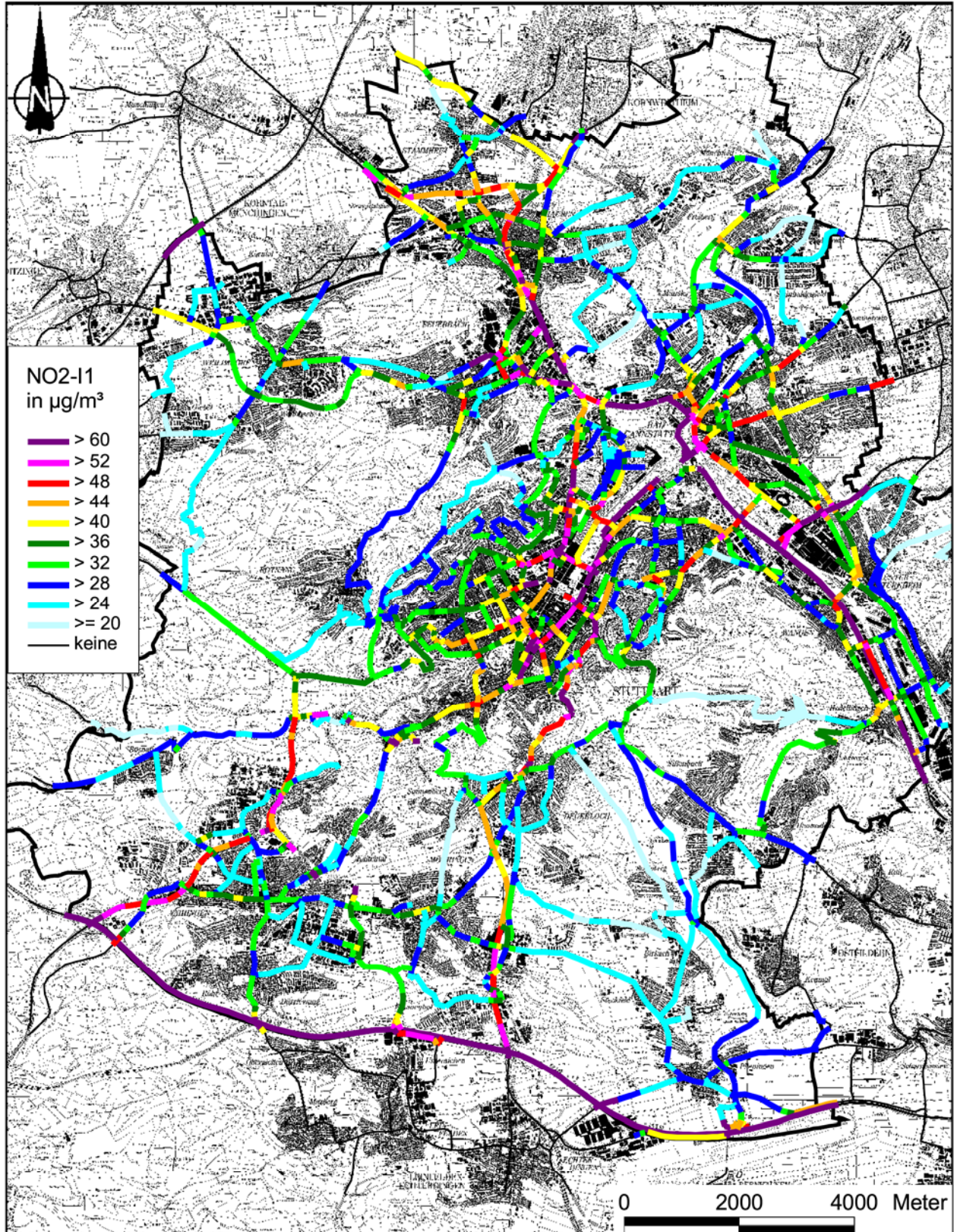
Abb. A2.1: NO 2 -Immission (Jahresmittelwert) für den Istzustand im Jahr 2010 für das Straßennetz im Stadtgebiet von Stuttgart
