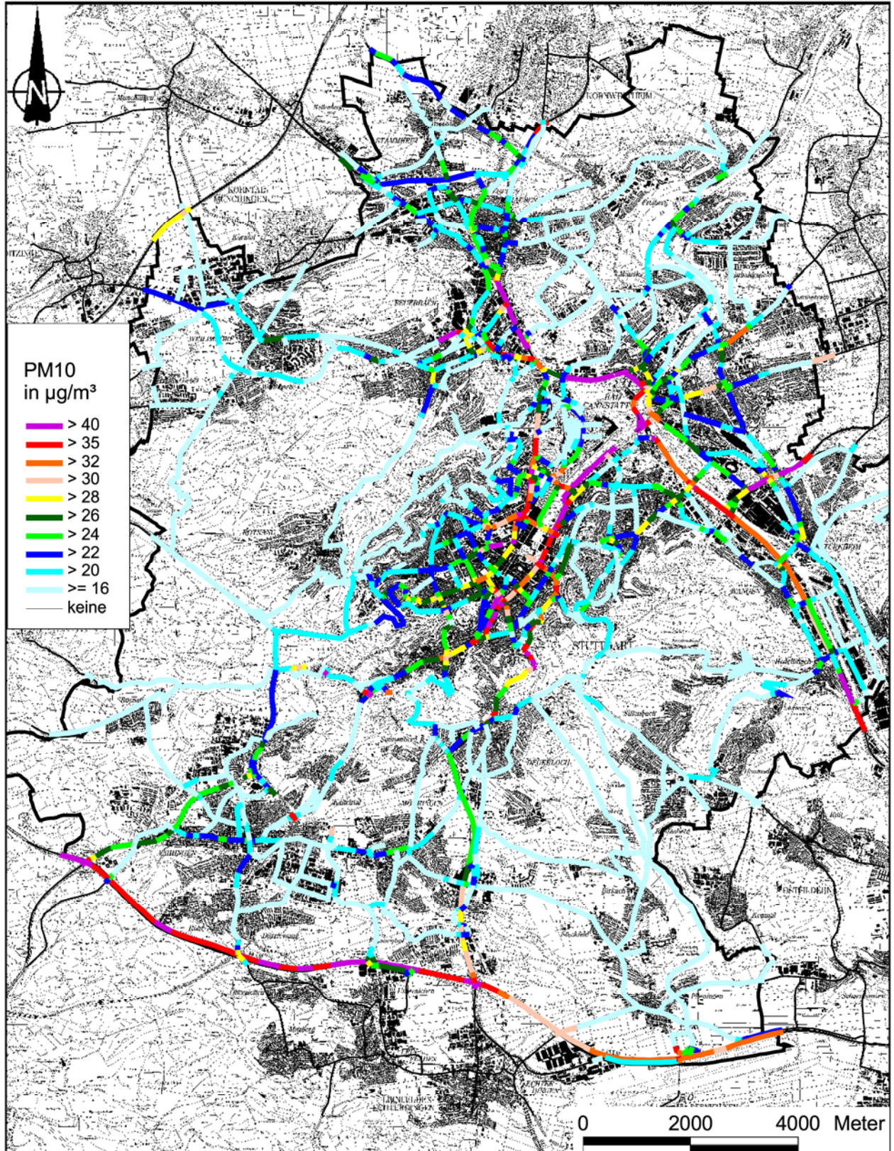
Abb. A2.4: PM10-Immission (Jahresmittelwert) für den Istzustand im Jahr 2010 für das Strassennetz im Stadtgebiet von Stuttgart
